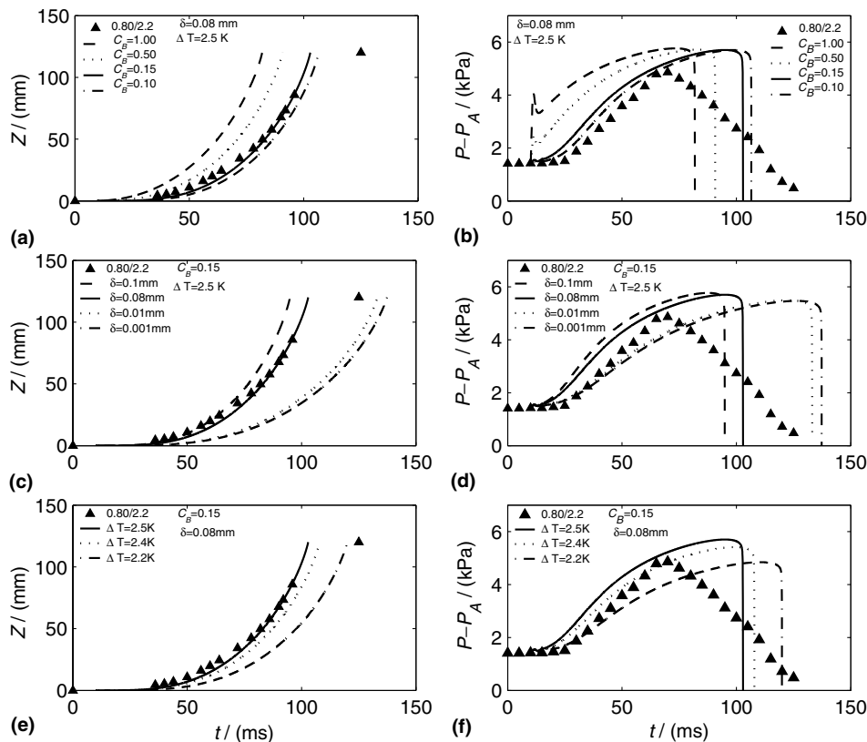
Fig. 7. Sensitivity of simulations to modelling parameters for run 0.80/2.2: (a), (b) C_B ; (c), (d) \delta ; (e), (f) \Delta T = T_0 - T_S(P_A) .
